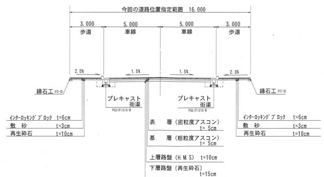
D-D' 断面図 1/200
