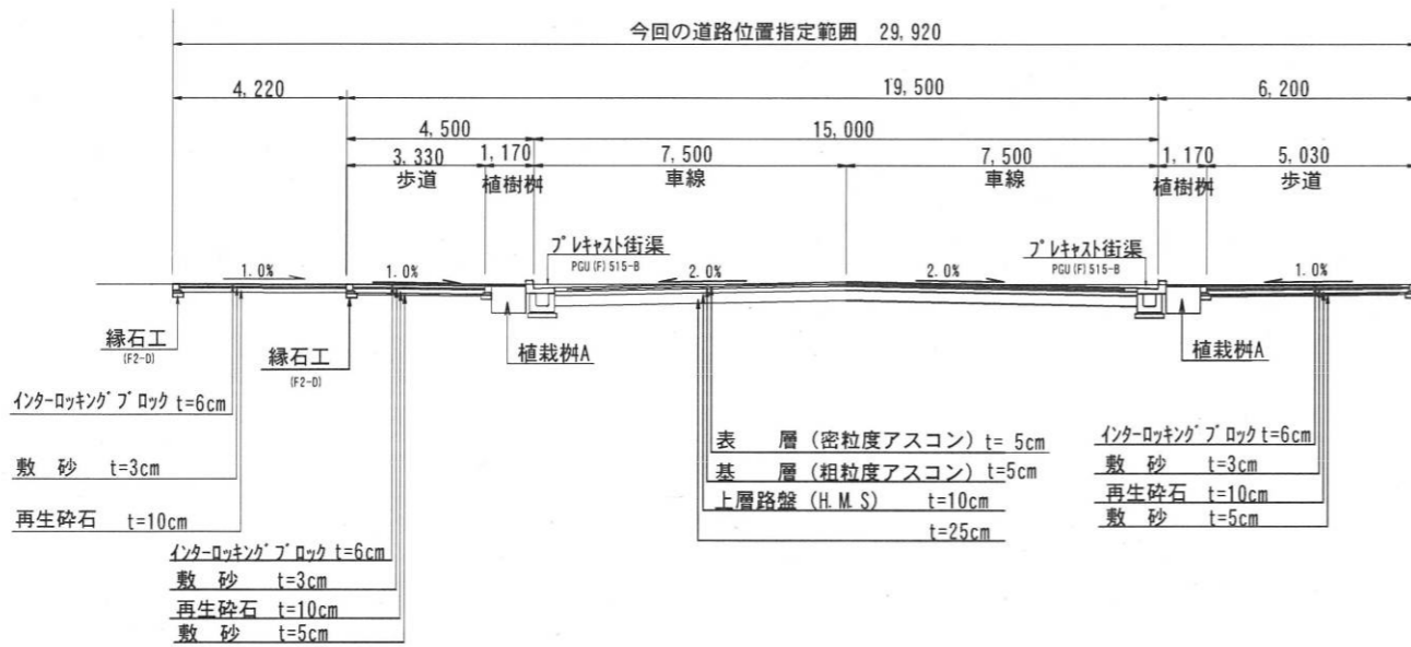
B-B' 断面図 1/200
