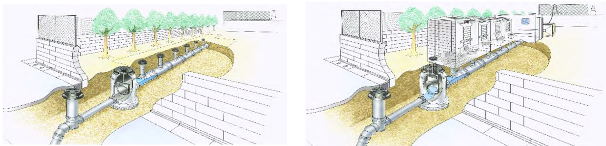
図 公共下水道接続型トイレ
