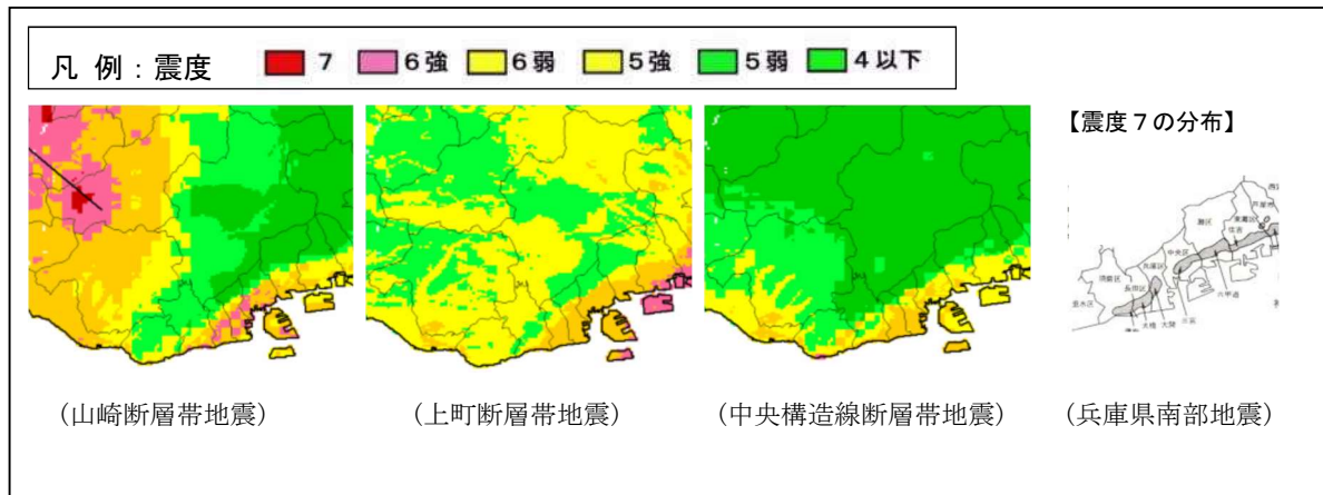
図 6-1-4 対象地震による震度分布
