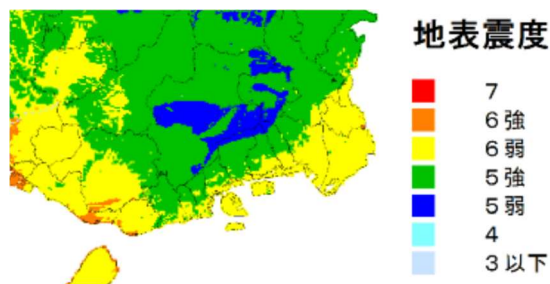
図6-1-8 地表震度分布
