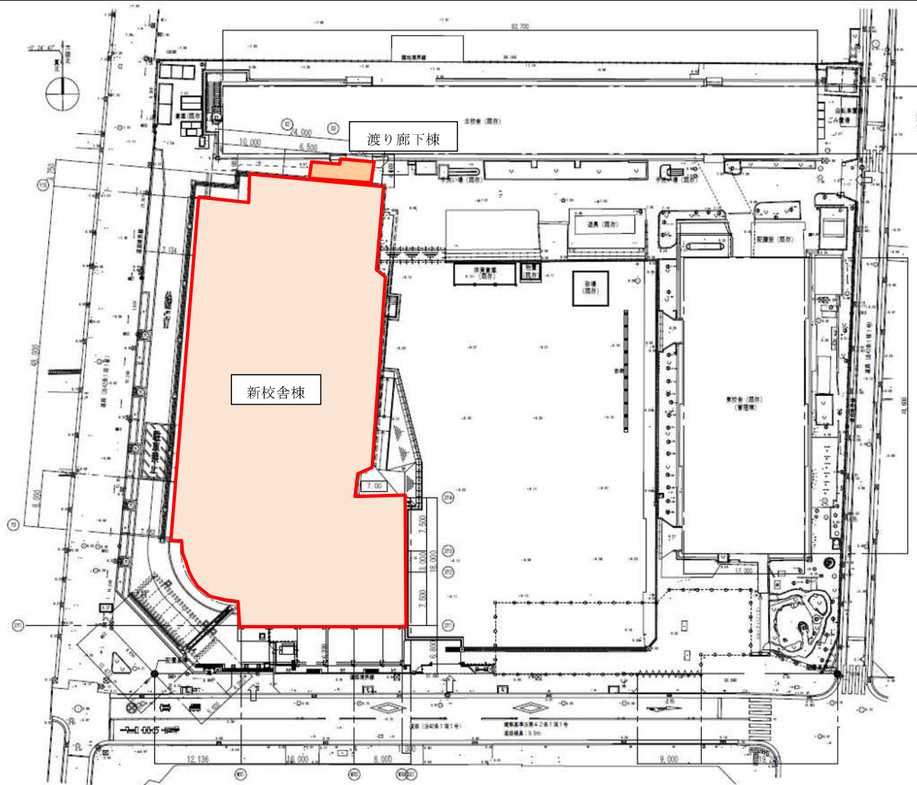
配置図
