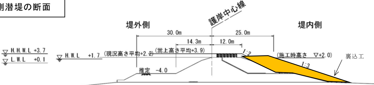
図 I -3-4 (2) 潜堤築造場所及び護岸築造場所の断面図
