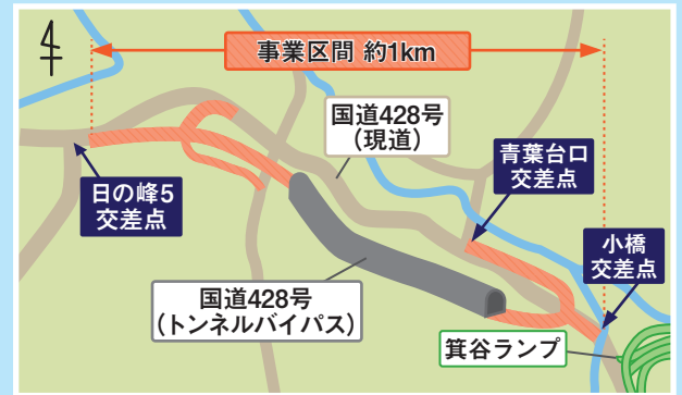
道路整備計画図
